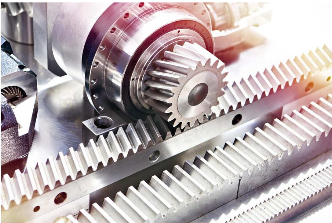
齿条齿轮传动系统 Rack & Pinion Drive Systems
